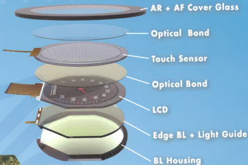
Standard Round LCD Edge Back Light
