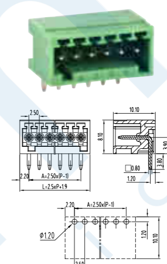
TLPHC-006R
