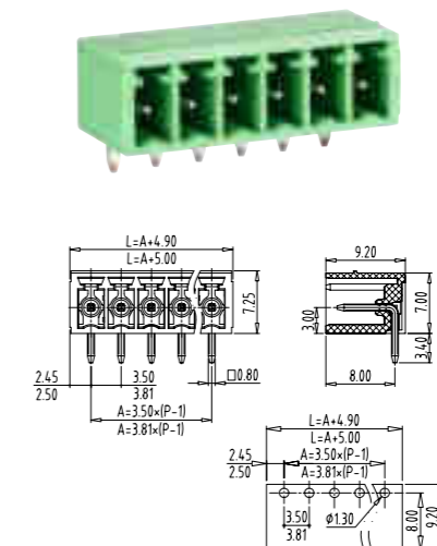
TLPHC-001R(TLPHC-100R)
