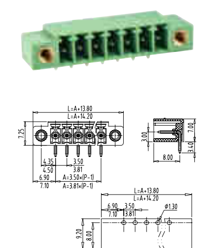
TLPHW-001R(TLPHW-100R)
