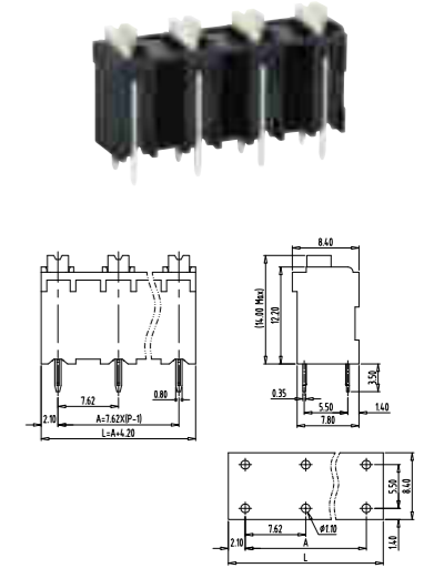
TLM-004VT-7.62
