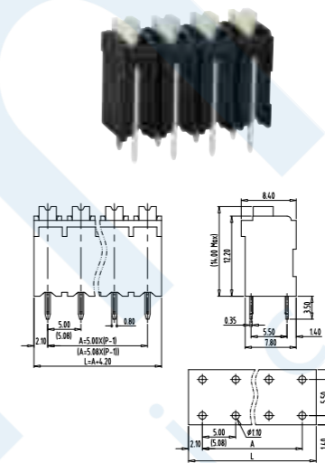
TLM-004VT-5.00(TLM-004VT-5.08)
