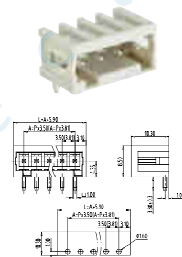
TLCH-001R(TLCH-100R)
