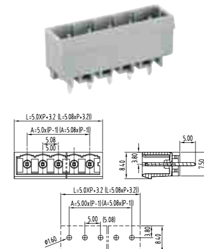
TLCH-200V(TLCH-300V)
