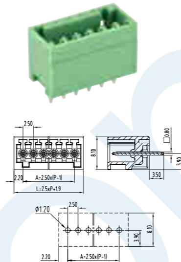
TLPHC-006V
